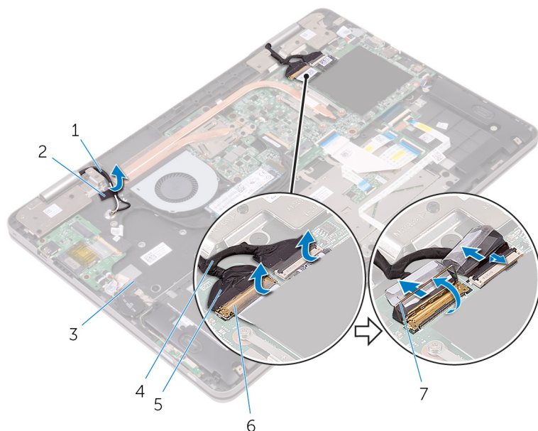
图 26: 断开电缆连接
