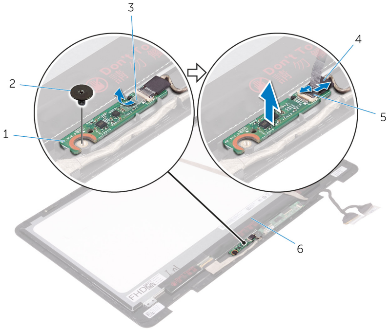
图 40: 卸下传感器板电缆
