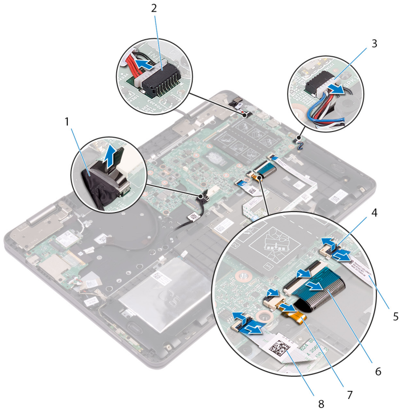
图 30: 断开电缆连接
