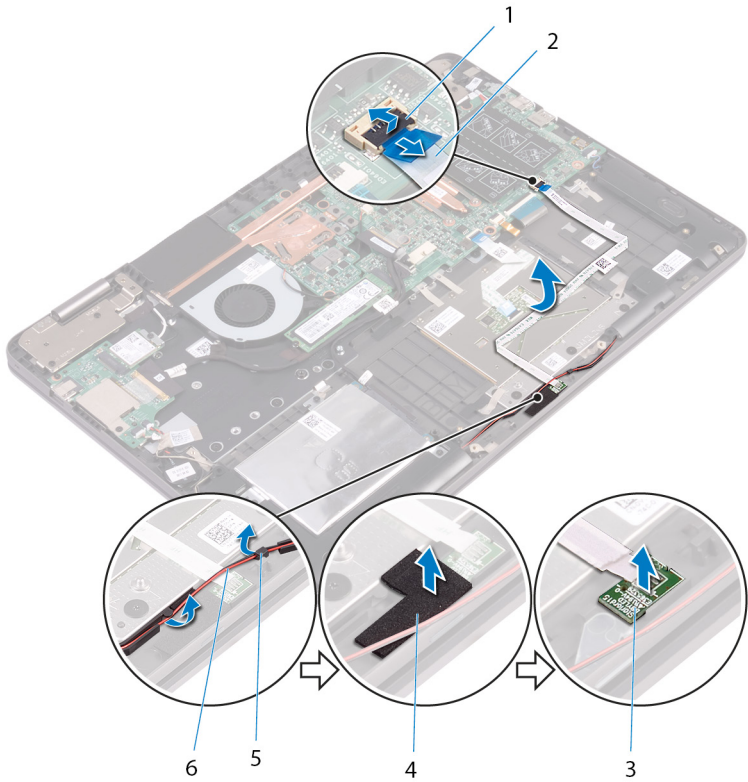
图 16: 卸下状态指示灯板
