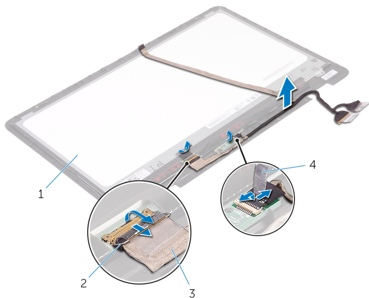
图 41: 卸下显示屏电缆
