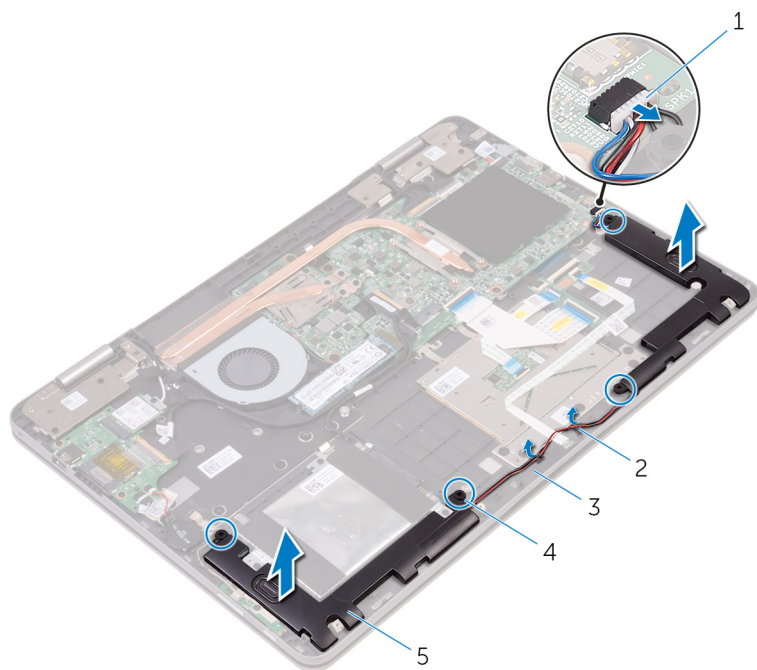
图 15: 卸下扬声器
