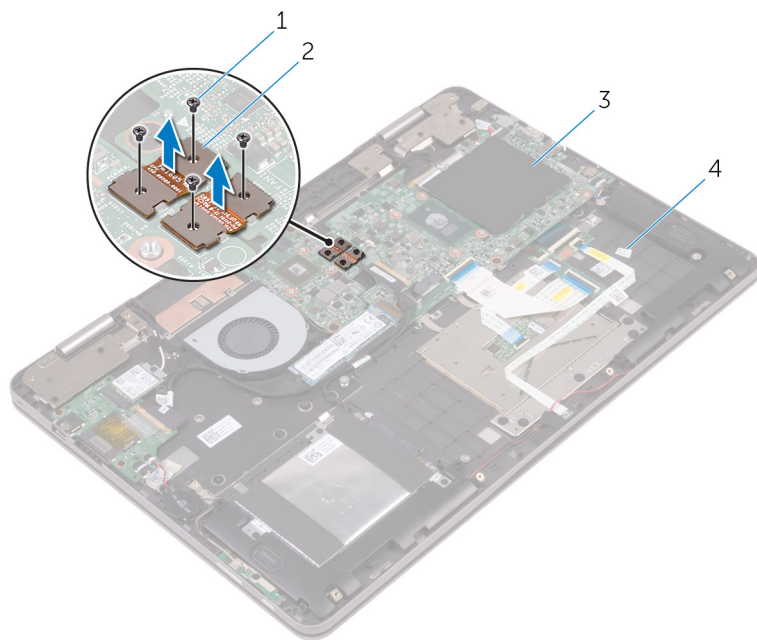
图 23: 卸下图形卡子板支架
