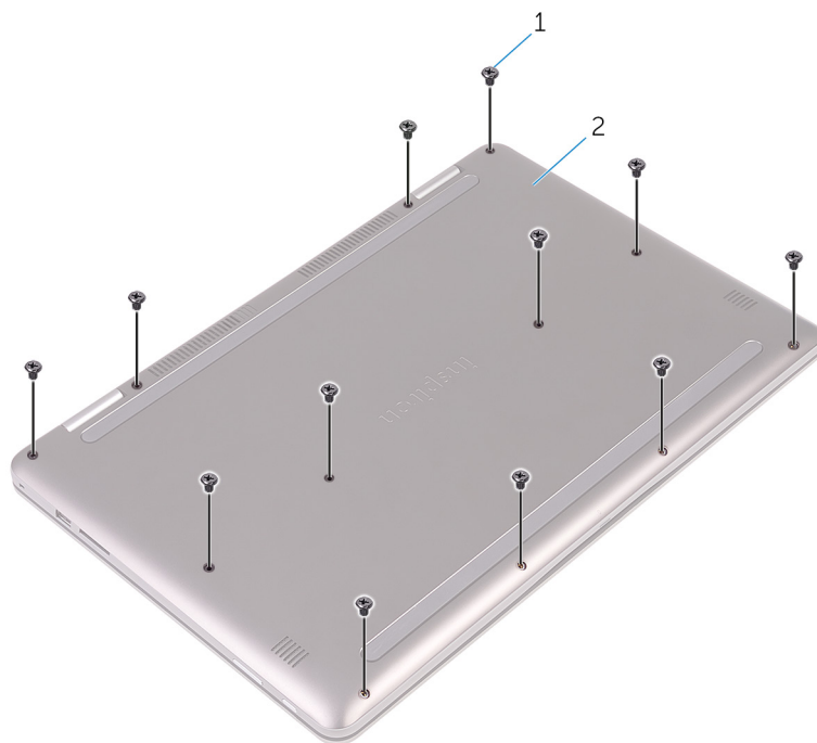
图 1: 拧下螺钉
