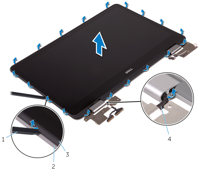
图 36: 卸下显示屏面板部件
