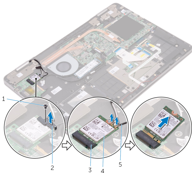
图 13: 卸下无线网卡
