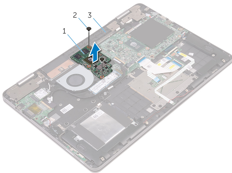
图 24: 卸下图形卡子板
