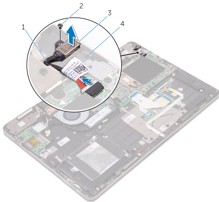
图 21: 卸下电源适配器端口
