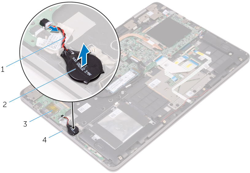
图 12: 取出币形电池
