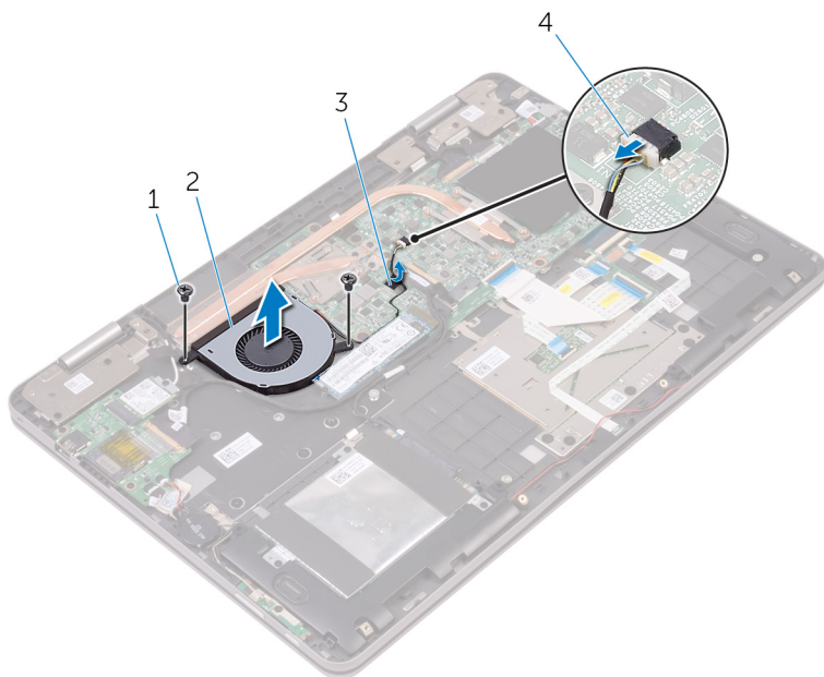
图 19: 卸下风扇
