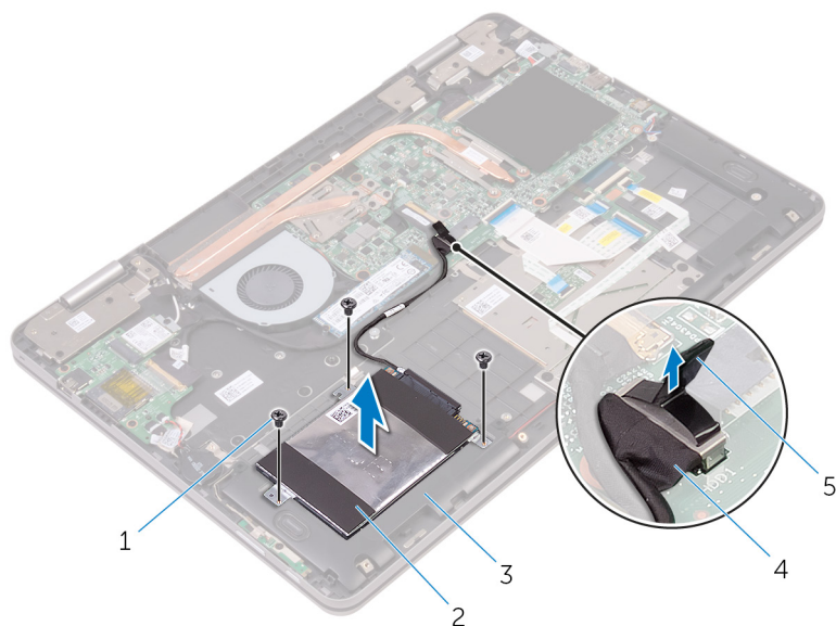
图 9: 卸下硬盘驱动器部件
