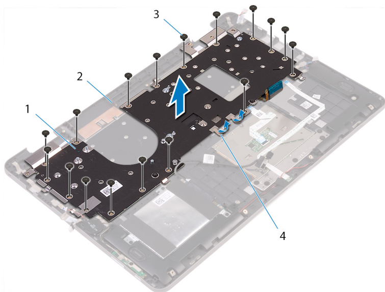
图 33: 卸下键盘支架
