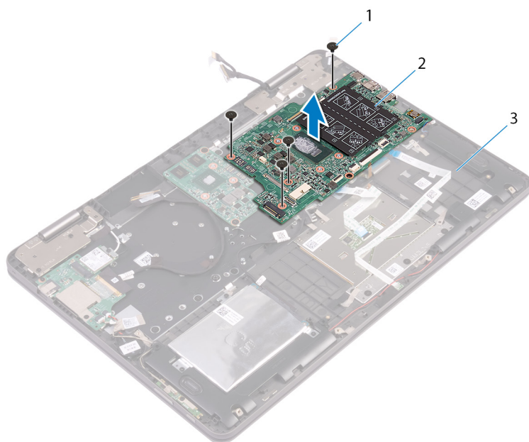
图 32: 卸下系统板
