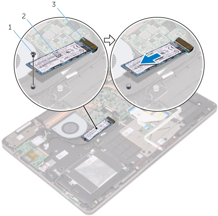
图 7: 卸下固态硬盘
