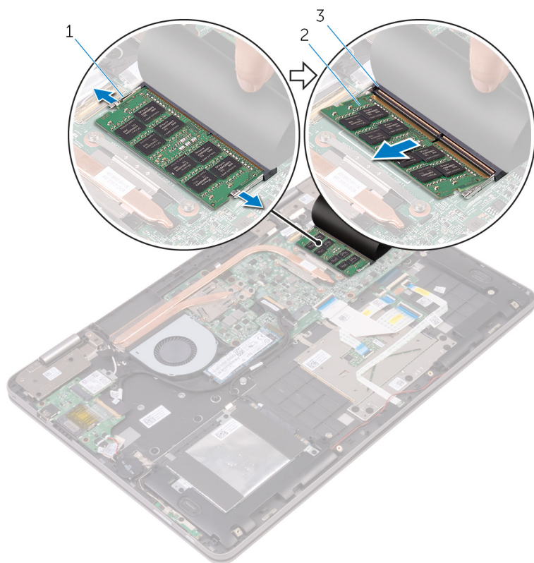
图 5: 卸下内存模块
