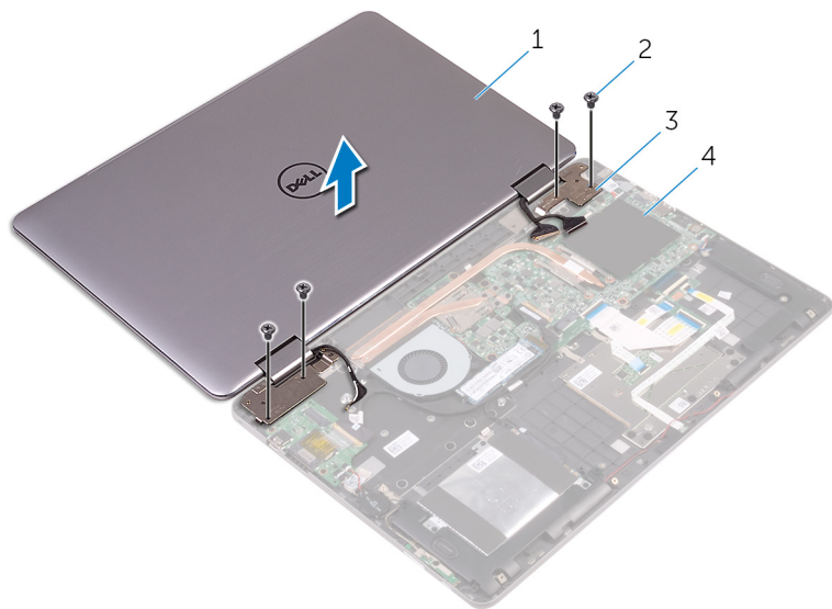
图 27: 卸下显示屏部件
