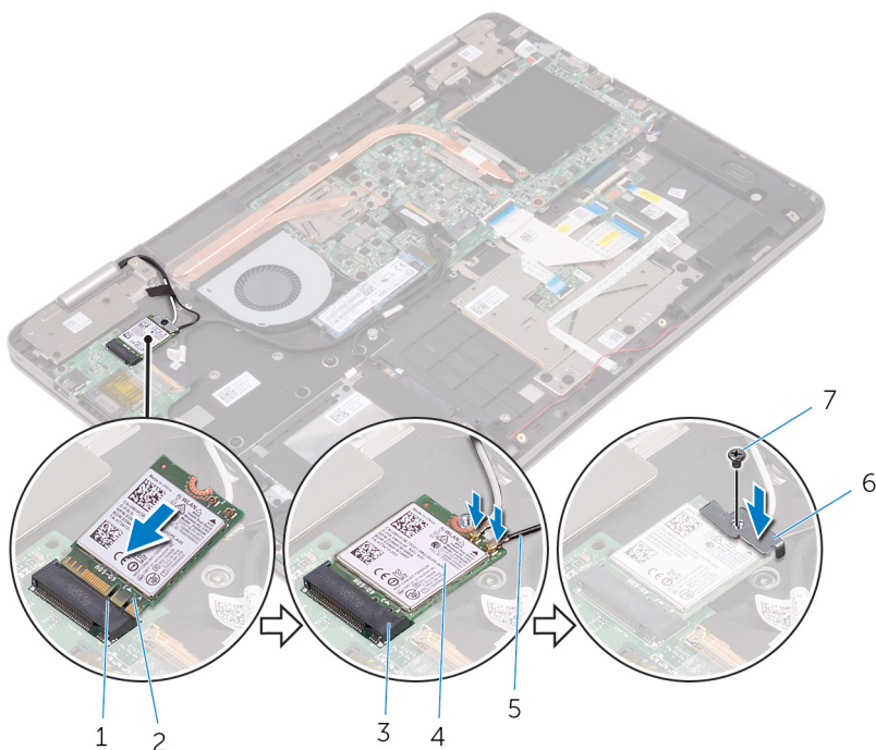
图 14: 装回无线网卡
