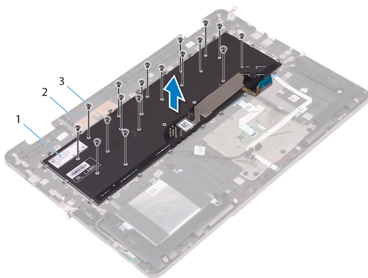
图 34: 卸下键盘
