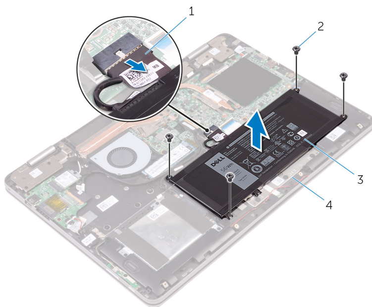
图 3: 卸下电池
