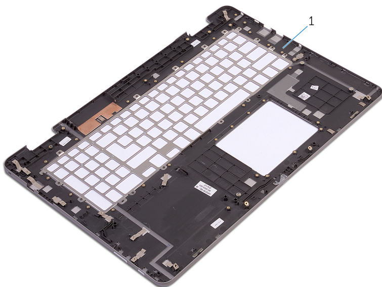
图 35: 卸下掌垫
