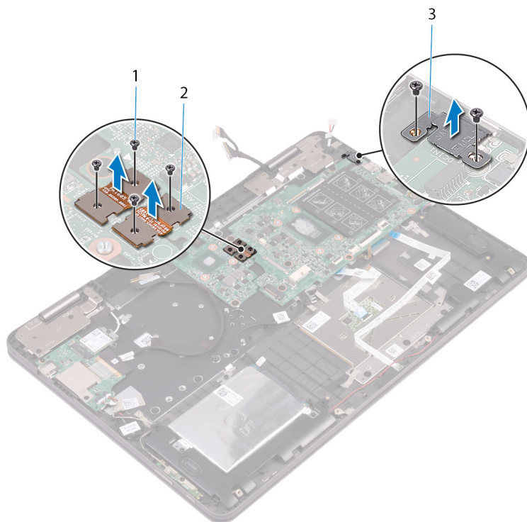
图 31: 卸下支架
