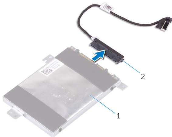
图 10: 卸下插入器
