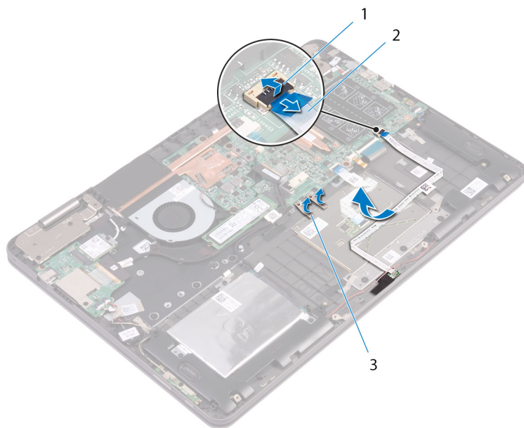
图 17: 卸下触摸板电缆
