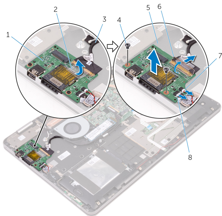
图 25: 卸下 I/O 板
