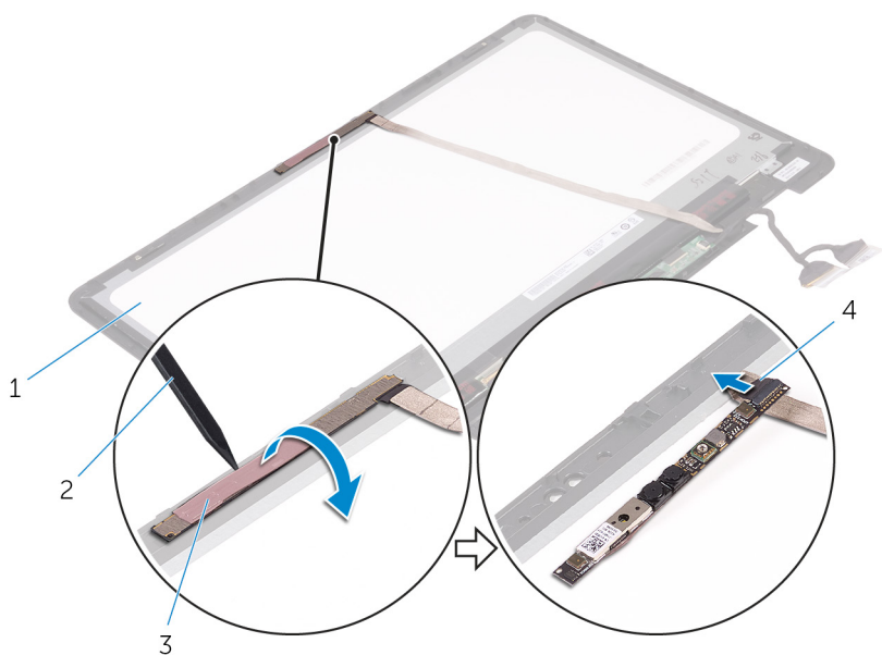
图 39: 卸下摄像头
