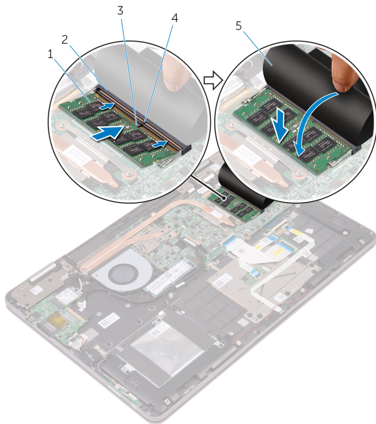
图 6: 装回内存模块
