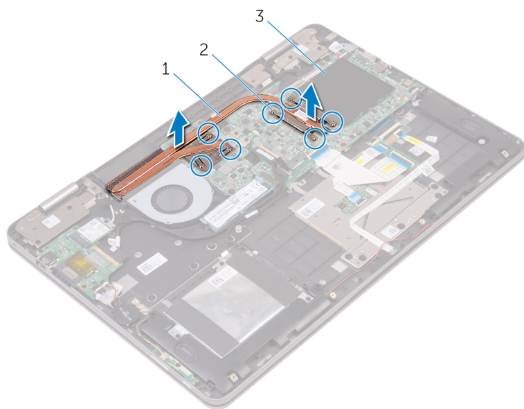
图 20: 卸下散热器
