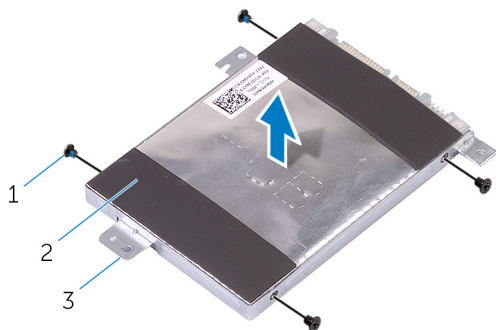
图 11: 卸下硬盘驱动器支架
