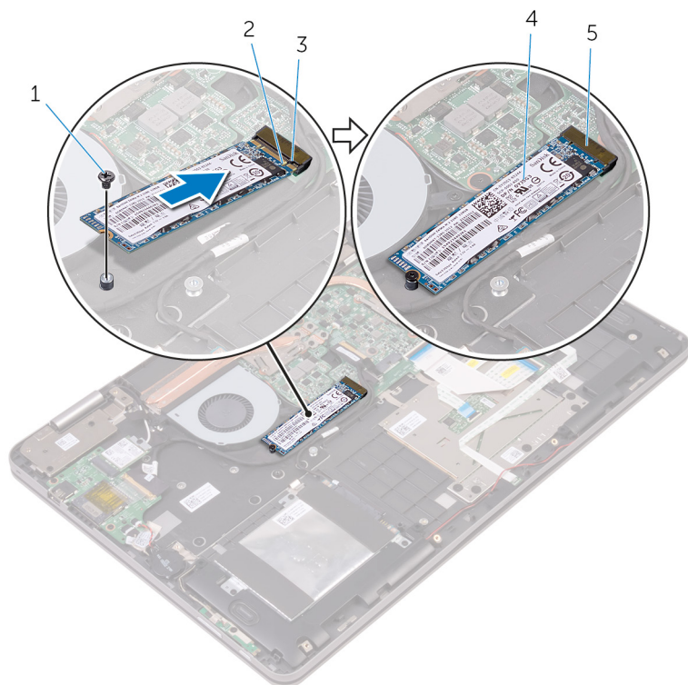
图 8: 装回固态硬盘
