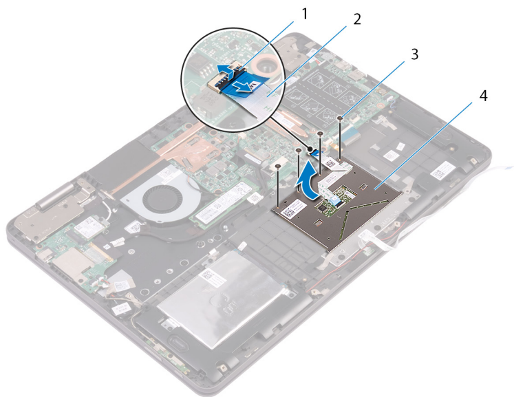
图 18: 卸下触摸板
