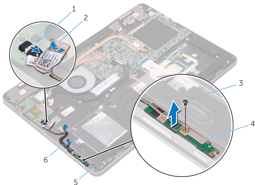
图 22: 卸下电源和音量按钮板
